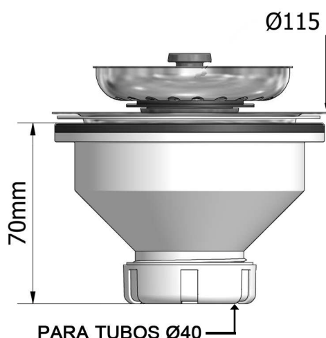
COTAS
